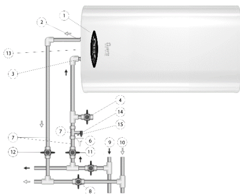
Малюнок 2. Схема підключення ЕВН до водопроводу в горизонтальному положенні
