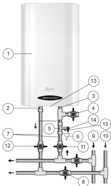
Малюнок 1. Схема підключення ЕВН до водопроводу в вертикальному положенні
