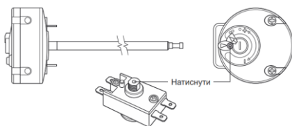
Малюнок 2. Можливі схеми розташування кнопки термовимикача. Термовимикач знаходиться під захисною кришкою
