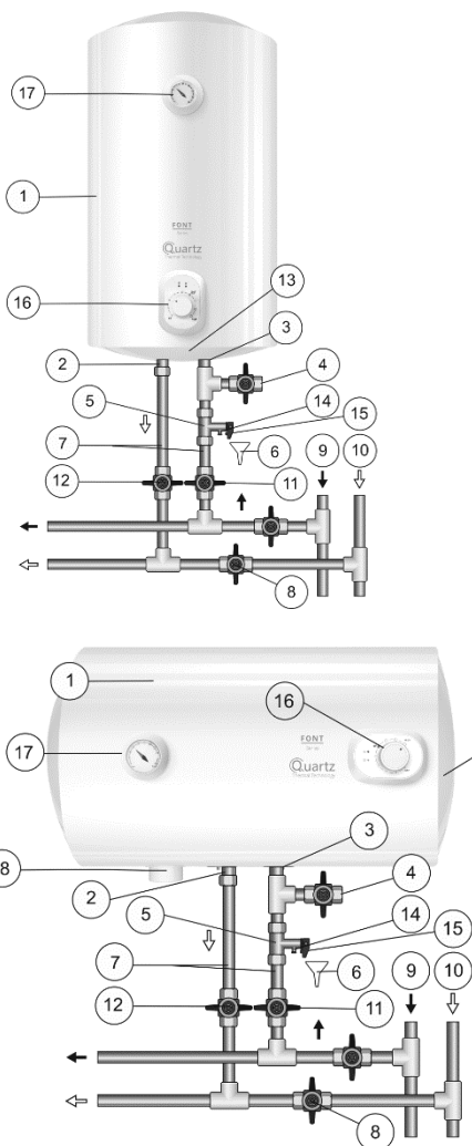
Малюнок 1. Схема підключення ЕВН до водопроводу
