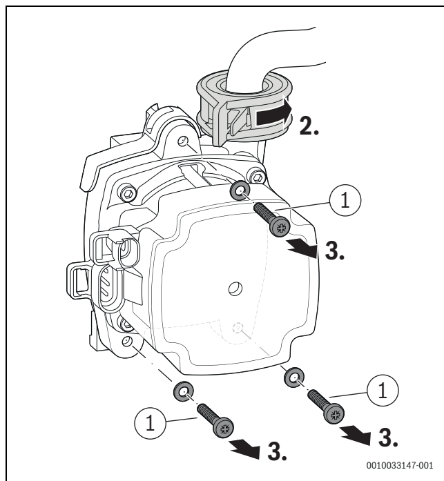
Мал. 68 Розблокуйте насос опалювального контуру та зніміть гвинти
