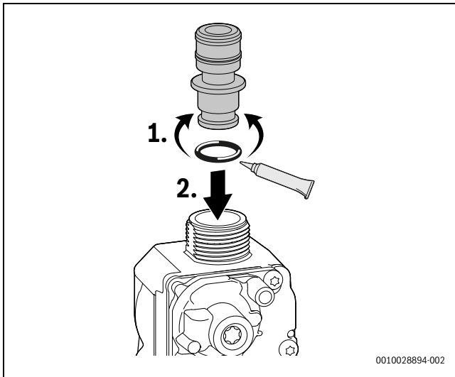
Мал. 77 Встановлення газового дрoселя
