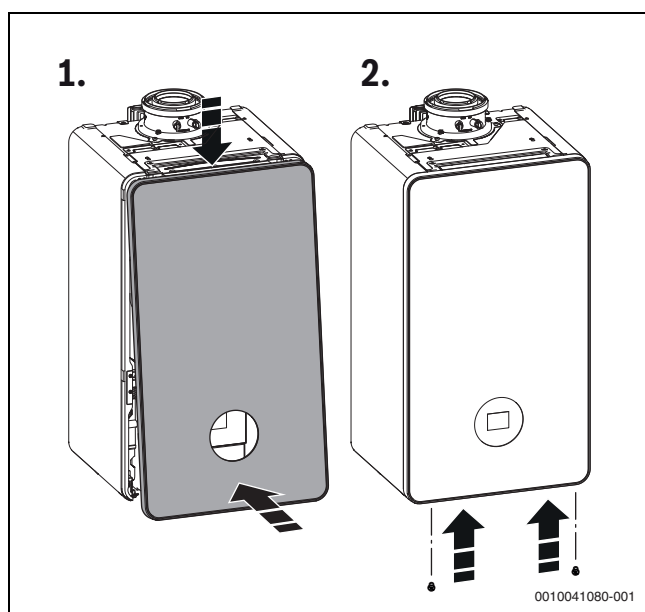
Мал. 40 Монтаж кожуха
