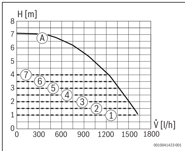
Мал. 89 Характеристики насоса та криві характеристик насоса
