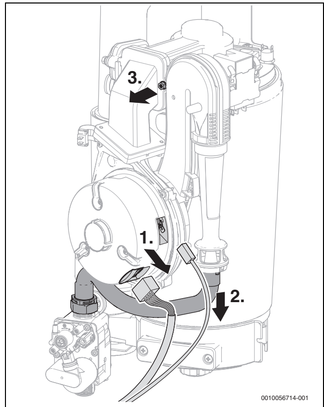
Мал. 52 Знімання штекера і газового шланга, відпускання гвинта
