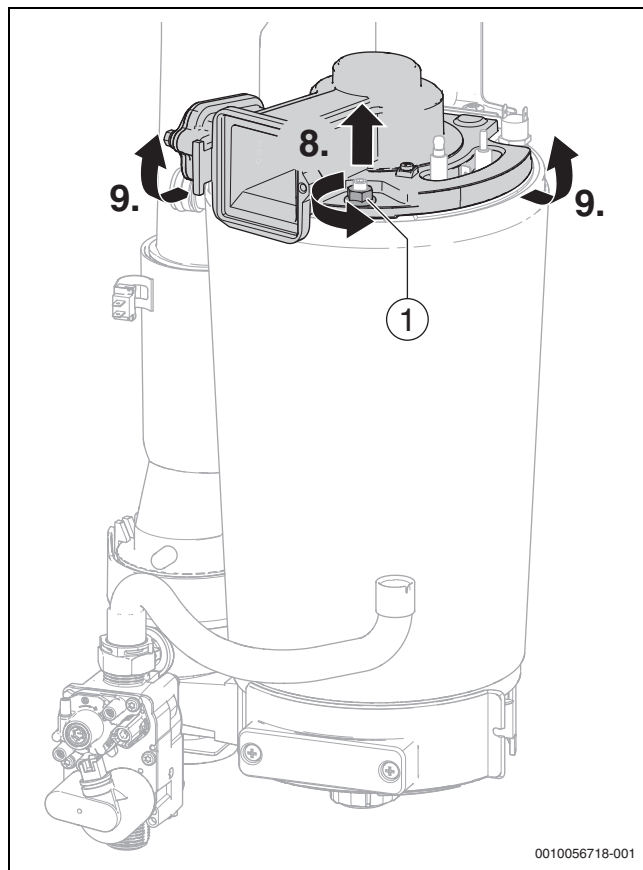
Мал. 55 Знімання кришки пальника разом з вентилятором та змішувальною камерою
