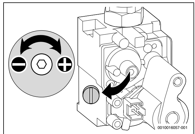
Мал. 45 Регулювання газової арматури
