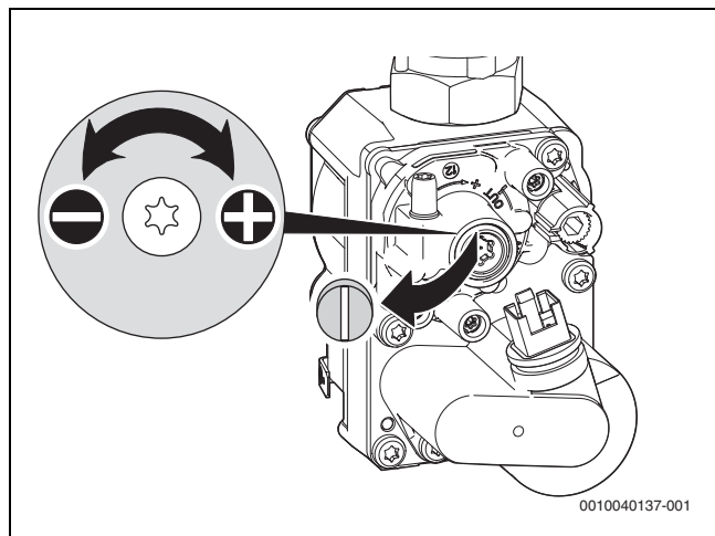
Мал. 46 Видалення пломби на регулювальному гвинті
