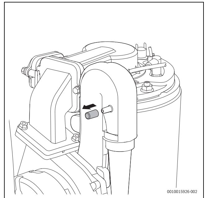
Мал. 50 Штуцер для вимірювання на змішувальній камері
