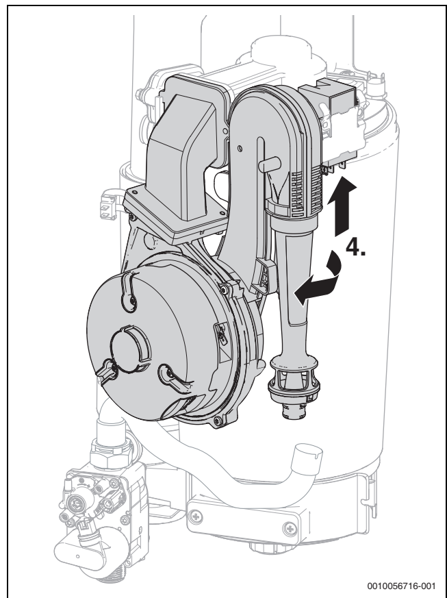
Мал. 53 Знімання трубки Вентурі зі змішувальною камерою та вентилятором
