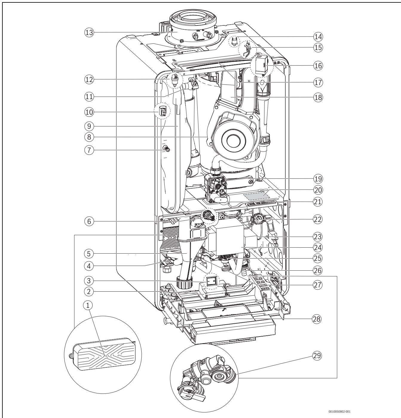
Мал. 6 Огляд виробу, двоконтурний котел
