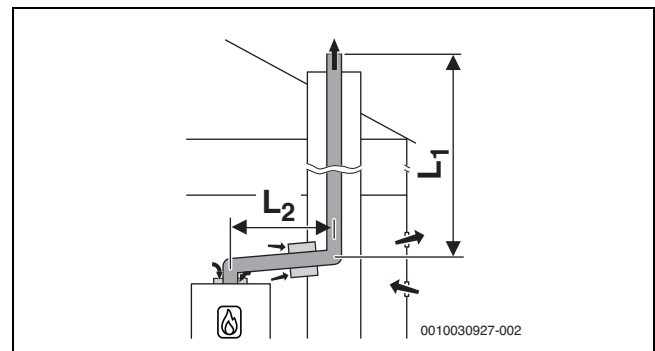
Мал. 19 Система відведення димових газів у шахті жорсткої конструкції відповідно до B 53p з подачею повітря у прилад з приміщення та концентричною з'єднувальною деталлю між котельним приміщенням та шахтою
