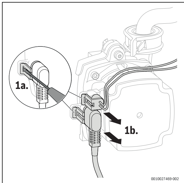
Мал. 67 Зніміть штекер з насоса опалювального контуру
