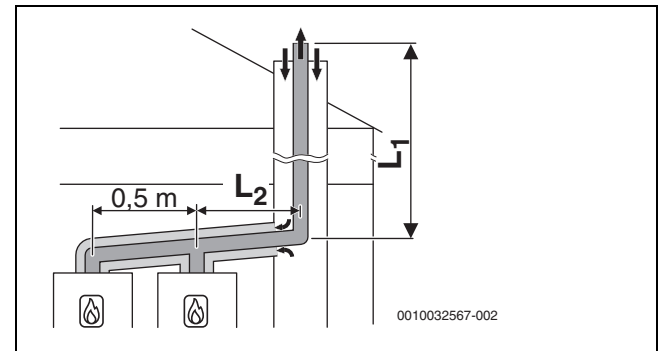
Мал. 24 Каскад з 2 приладами:
