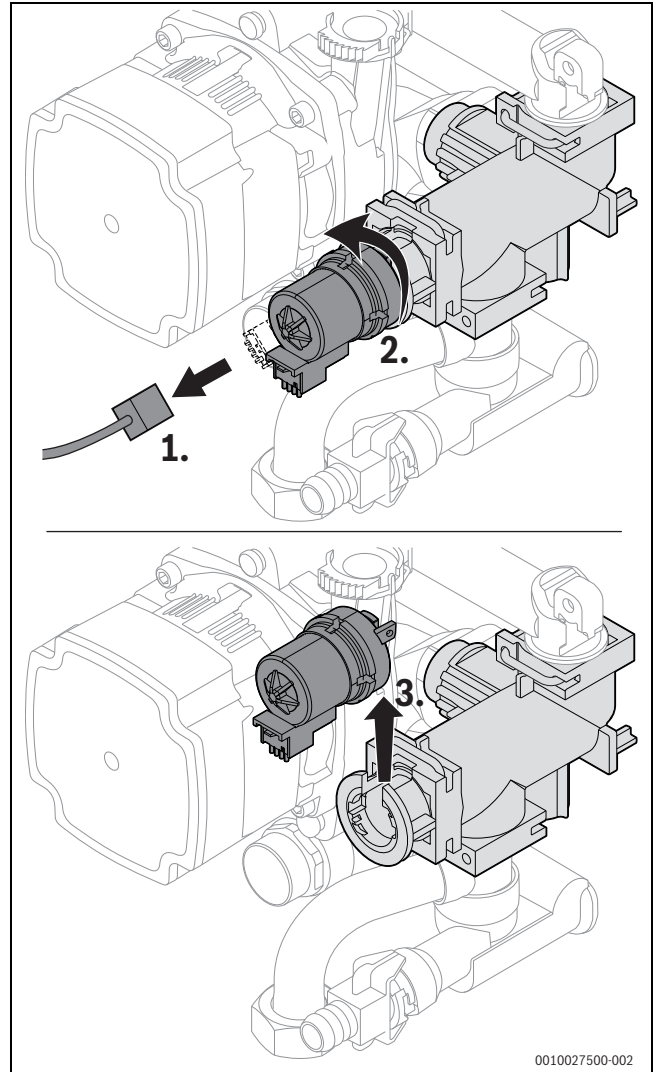
Мал. 85 Демонтаж двигуна 3-ходового клапана (варіант без гвинтів)
