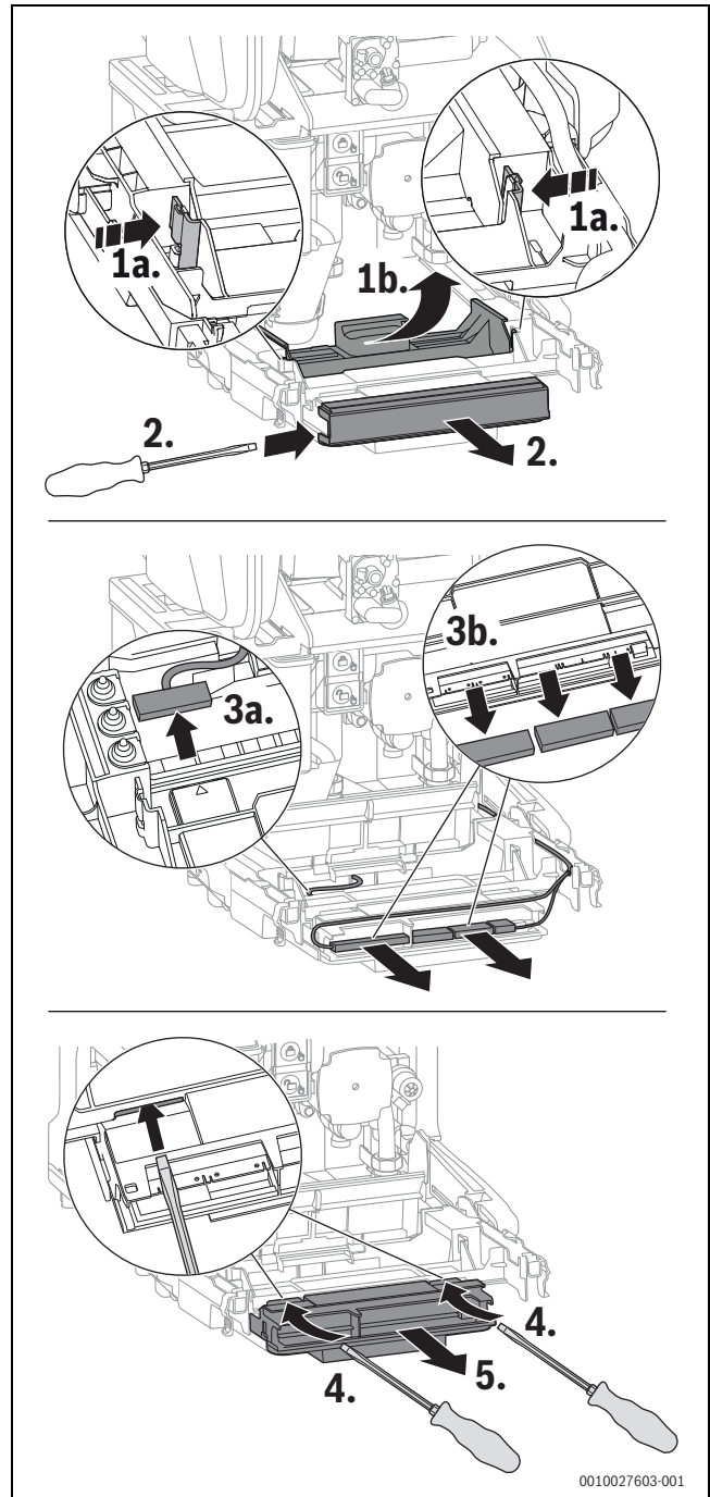
Мал. 79 Витягніть систему керування
