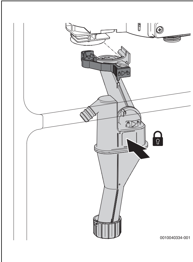
Мал. 84 Встановлення сифона для відведення конденсату
