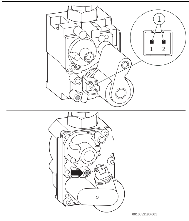
Мал. 51 Точки вимірювання на газовій арматурі
