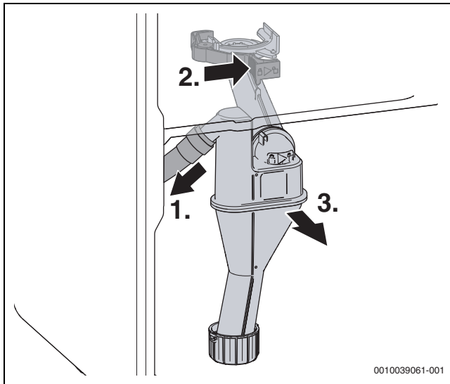
Мал. 80 Демонтаж сифона для конденсату
