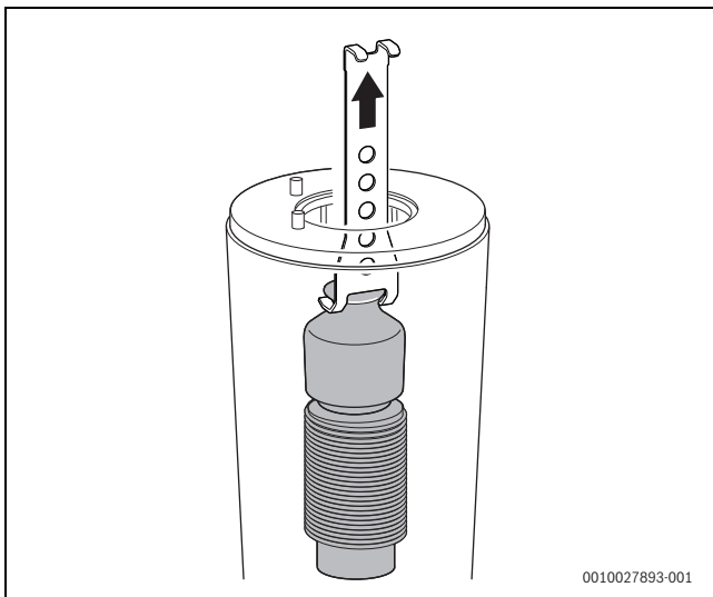
Мал. 57 Виймання верхнього елемента теплообмінника, що служить для оптимізації розподілювання тепла
