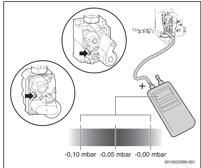
Мал. 44 Вимірювання різниці тиску
