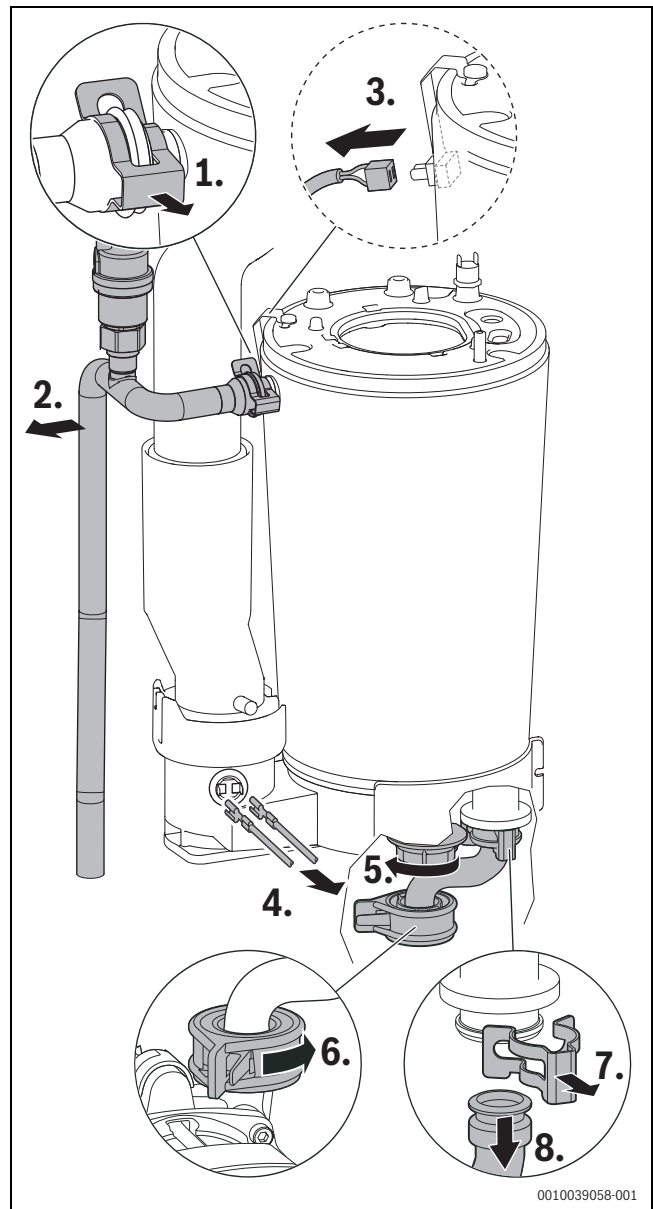
Мал. 65 Від'єднання труби лінії подачі, зняття кабелю та зняття труби зворотної лінії
