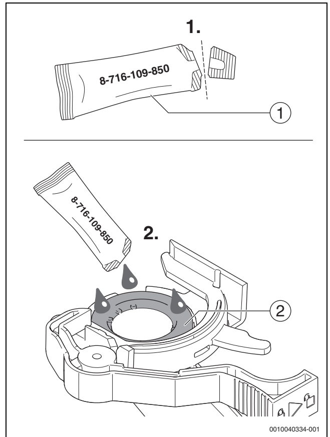
Мал. 83 Змащення ущільнення
