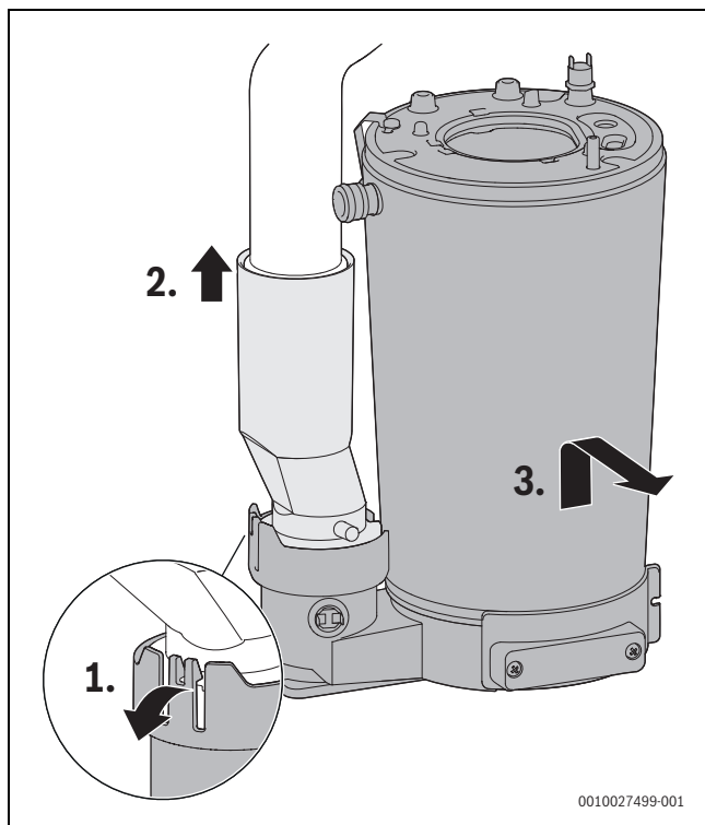
Мал. 66 Демонтаж котлового блоку, який включає камеру згоряння і теплообмінник
