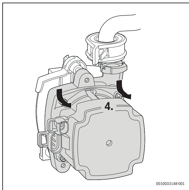
Мал. 69 Знімання насоса опалювального контуру
