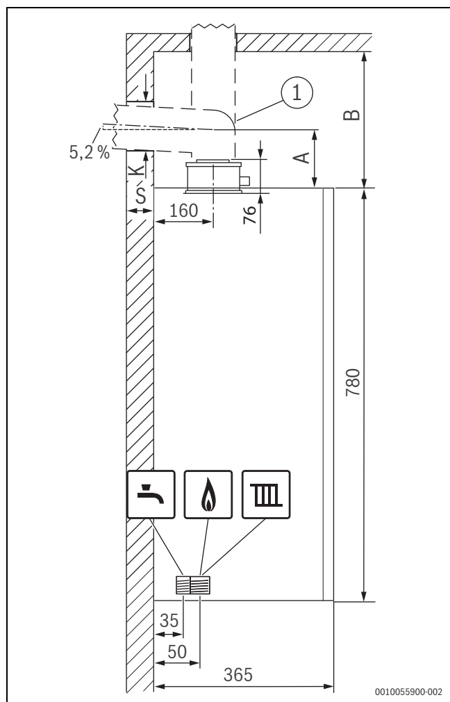
Мал. 2 Вигляд збоку (мм)
