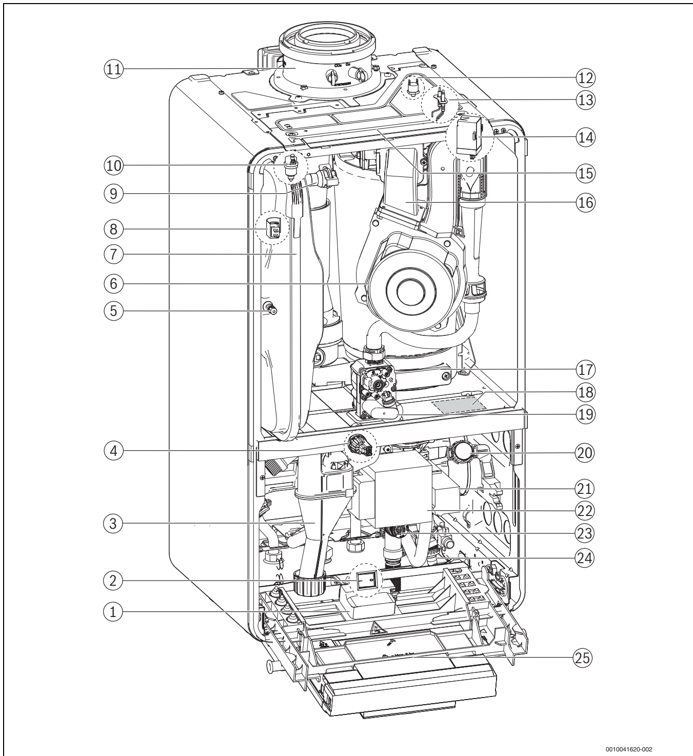
Мал. 7 Огляд виробу, бак непрямого нагріву
