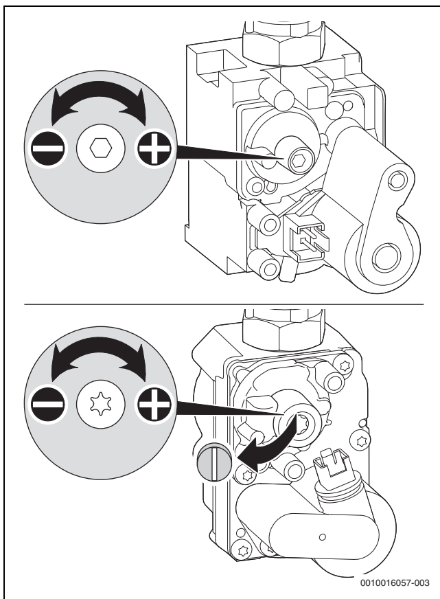
Мал. 48 Регулювання газової арматури
