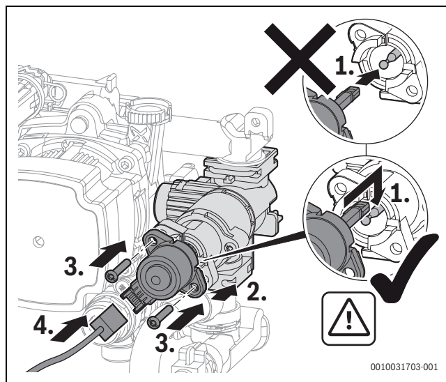
Мал. 88 Монтаж двигуна 3-ходового клапана (варіант з гвинтами)
