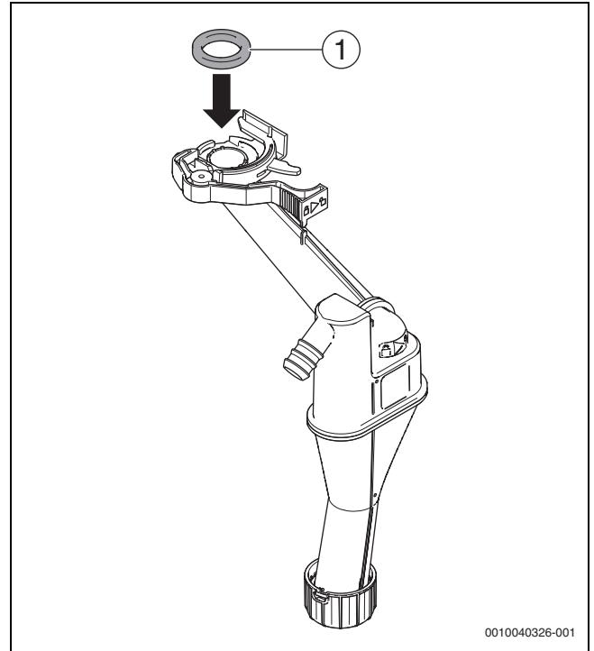
Мал. 82 Встановлення нового ущільнення на сифон для відведення конденсату
