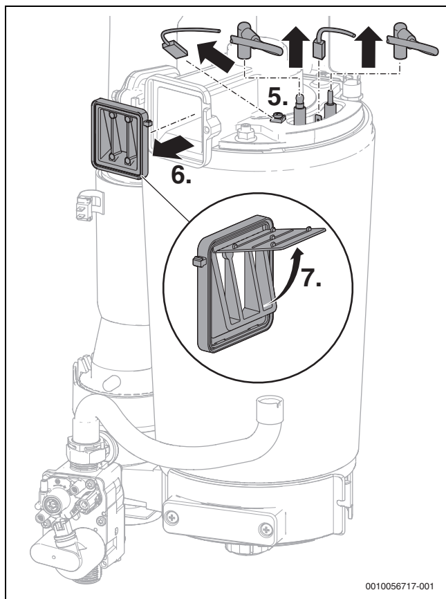
Мал. 54 Знімання кабелів
