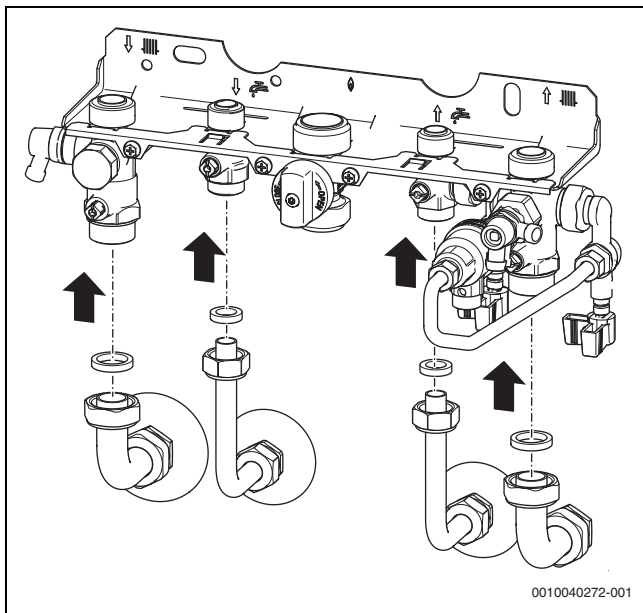
Мал. 29 Монтаж труб з ущільненнями на монтажну приєднувальну панель (додаткові комплектуючі)
