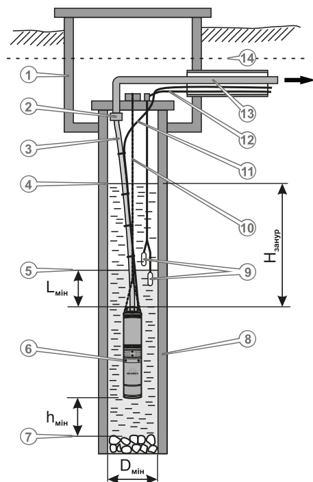
Рисунок 5. Схема монтажу насоса свердловинного.
