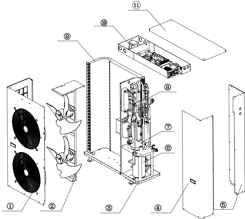
Експлозивна діаграма для BLN-015TA1/TA3, BLN-018TA1/TA3, BLN-026TA1/TA3, BLN-032TA1/TA3
